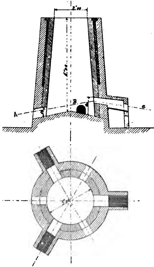
Fig. 161 et 162. — Four à cuire l'argile.
